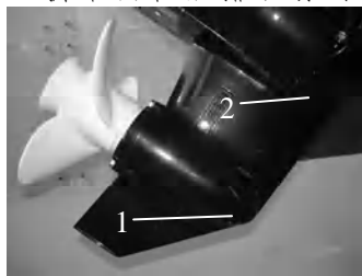
1. 放油螺钉 2. 油位孔塞
