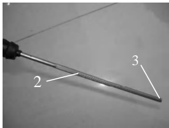
1. 油位尺 2. 高位标记 3. 低位标记
